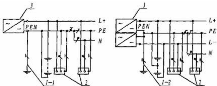
Рис. 1.7.3. Система TN-C-S переменного (а) и постоянного (б) тока. Нулевой защитный и нулевой рабочий проводники совмещены в одном проводнике в части системы:
