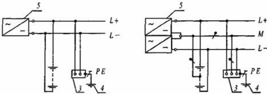
Рис. 1.7.4. Система IT переменного (а) и постоянного (б) тока. Открытые проводящие части электроустановки заземлены. Нейтраль источника питания изолирована от земли или заземлена через большое сопротивление:
